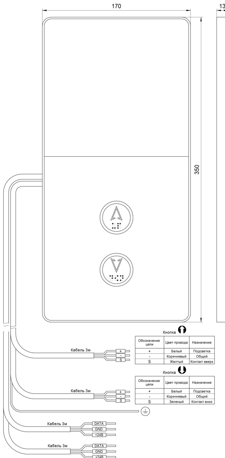
Рис.1 Внешний вид, габаритные и установочные размеры Вызывного поста МАЛАХИТ НШЕК.468381.077
